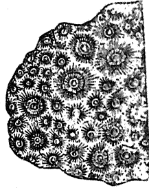
चित्र १६—काबोनिफेरस काल की मूँगे की भित्ति
